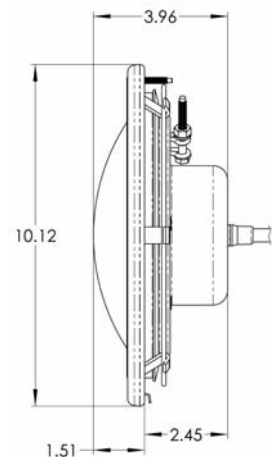
Dimensions
